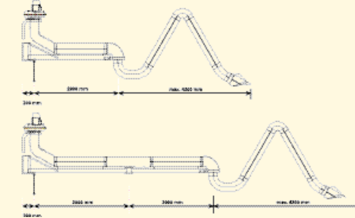
Reikwijdte van de NEC 2 en NEC 4 met (Ultra)Flex 4
